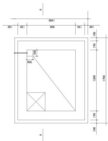
PŮDORYS
